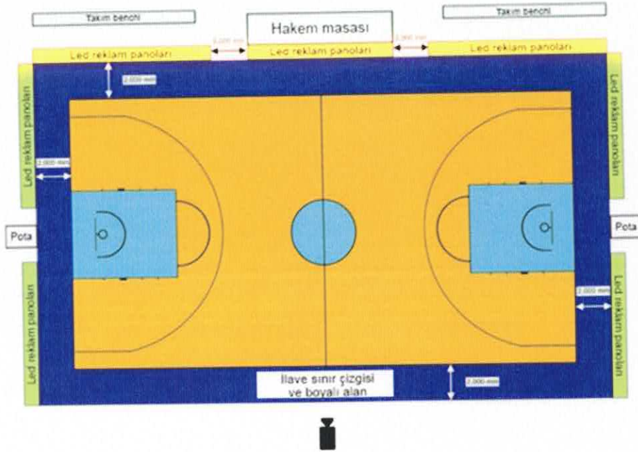
Çizim 14 Reklam panoları (Ana Kamera karşı tarafından)
