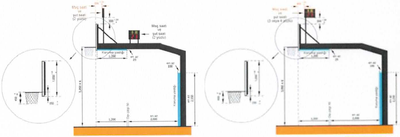
Çizim 6 Arkalık yerleşim alternatifleri
