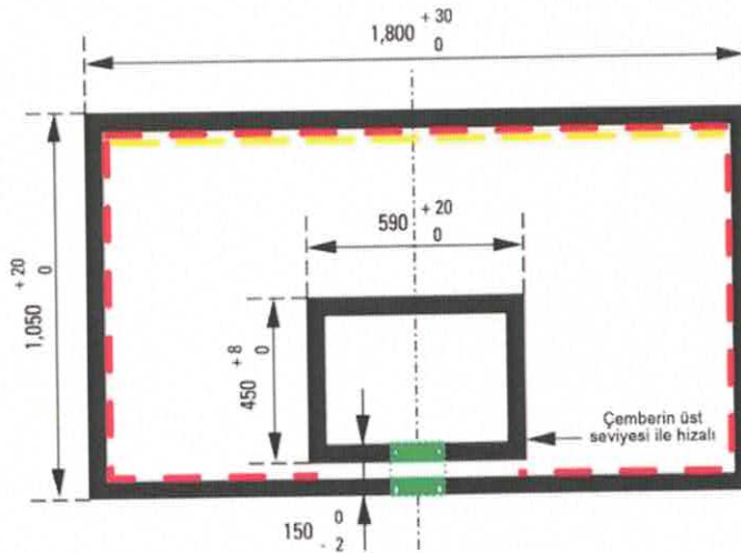
Çizim 5 Arkalık işaretleri
