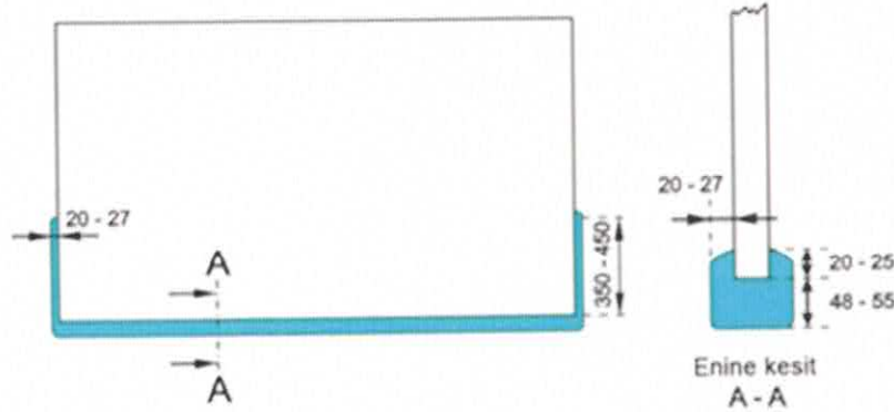
Çizim 7 Arkalık koruma yastığı
