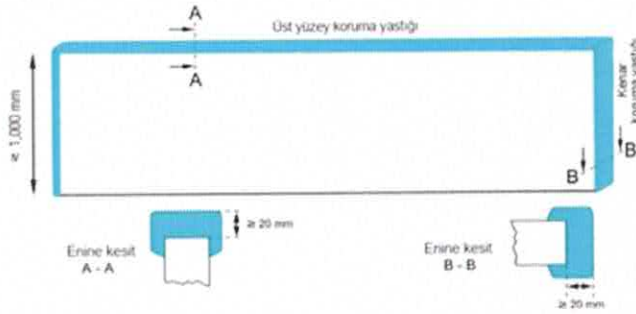
Çizim 15 Reklam panosu koruma yastığı
